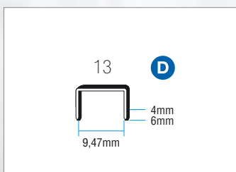
Μοντ. MART 13
