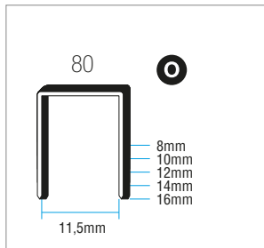
Μοντ. 80
