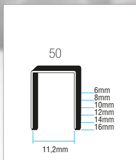
Μοντ. 50
