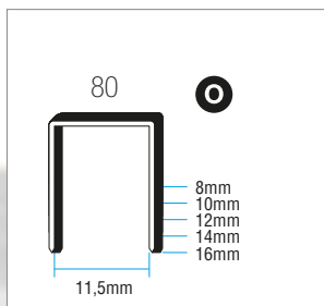
Μοντ. 80 Brad
