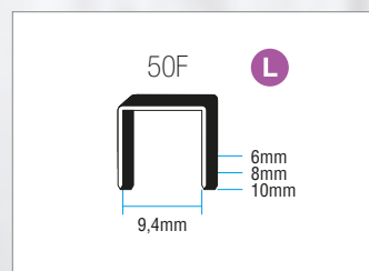
Μοντ. MART 50
